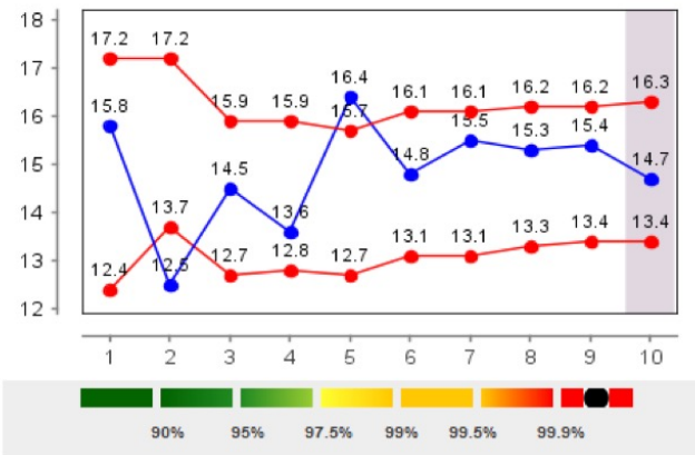
HGB
